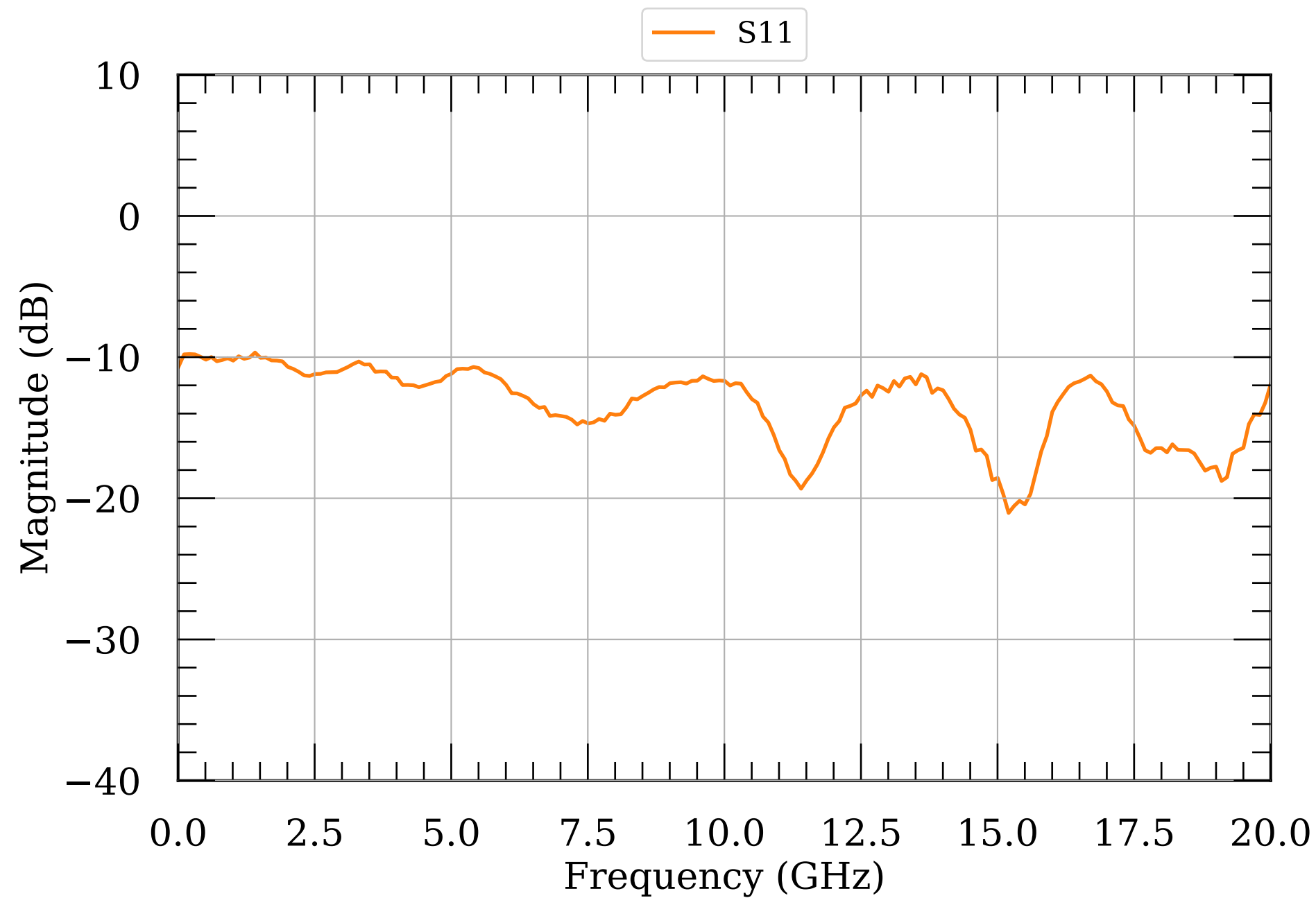
LNA S-params module030
